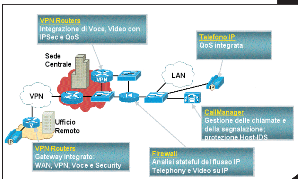
Figura 1. Schema generico di punti di protezione di una infrastruttura voce
