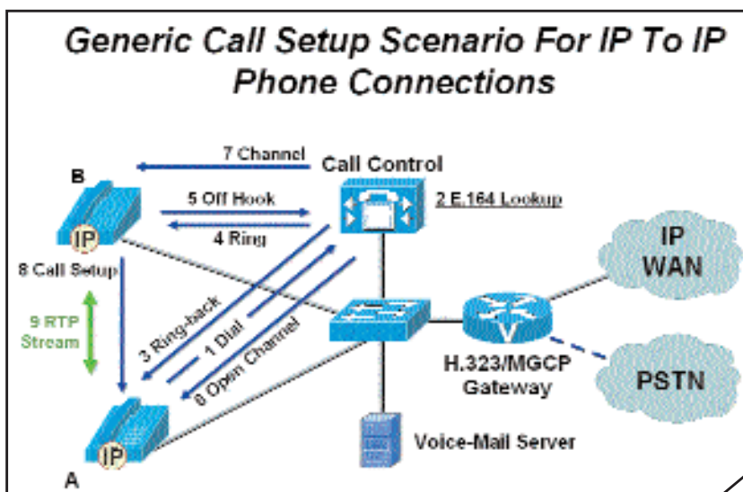
Figura 2. Processo di una chiamata IP
